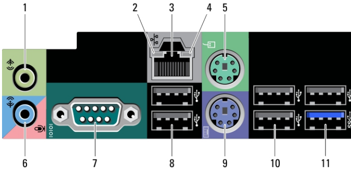
圖 2. 背面板視圖
